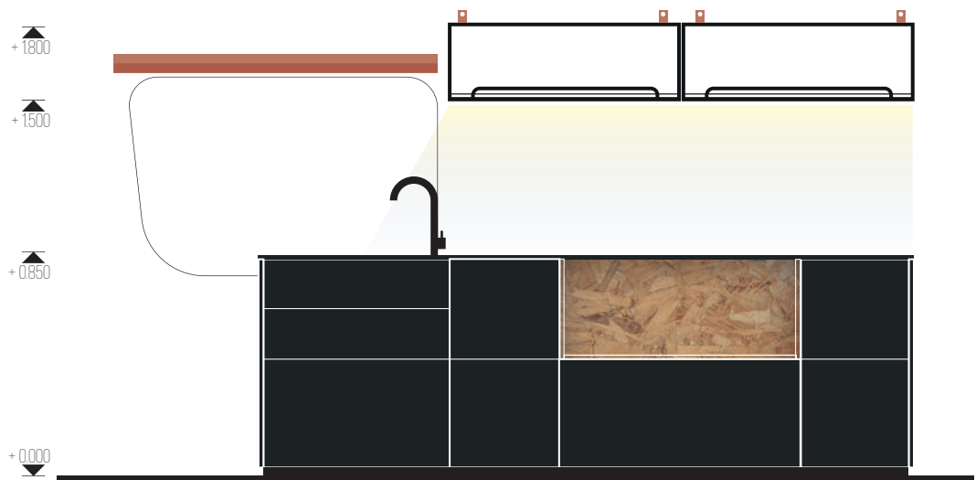
ANSICHT SEITE RECHTS
